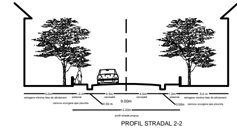
Profil Stradal Propus 2-2
