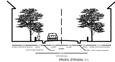
Profil Stradal Propus 1-1
